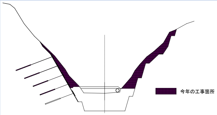
グラウンドアンカーを4段施工しました。
