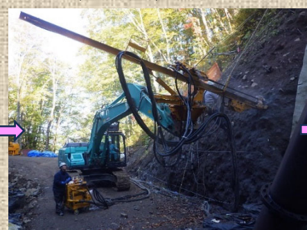
法面工（鉄筋挿入）
